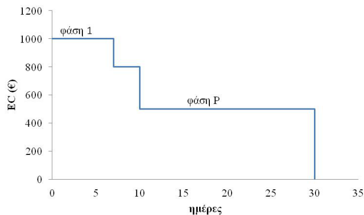
Σχήμα 3: Ενδεικτικό διάγραμμα πρόσθετου κυκλοφοριακού κόστους συναρτήσει του χρόνου
